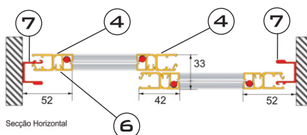
Secção Horizontal
