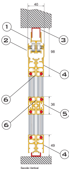
Secção Vertical
